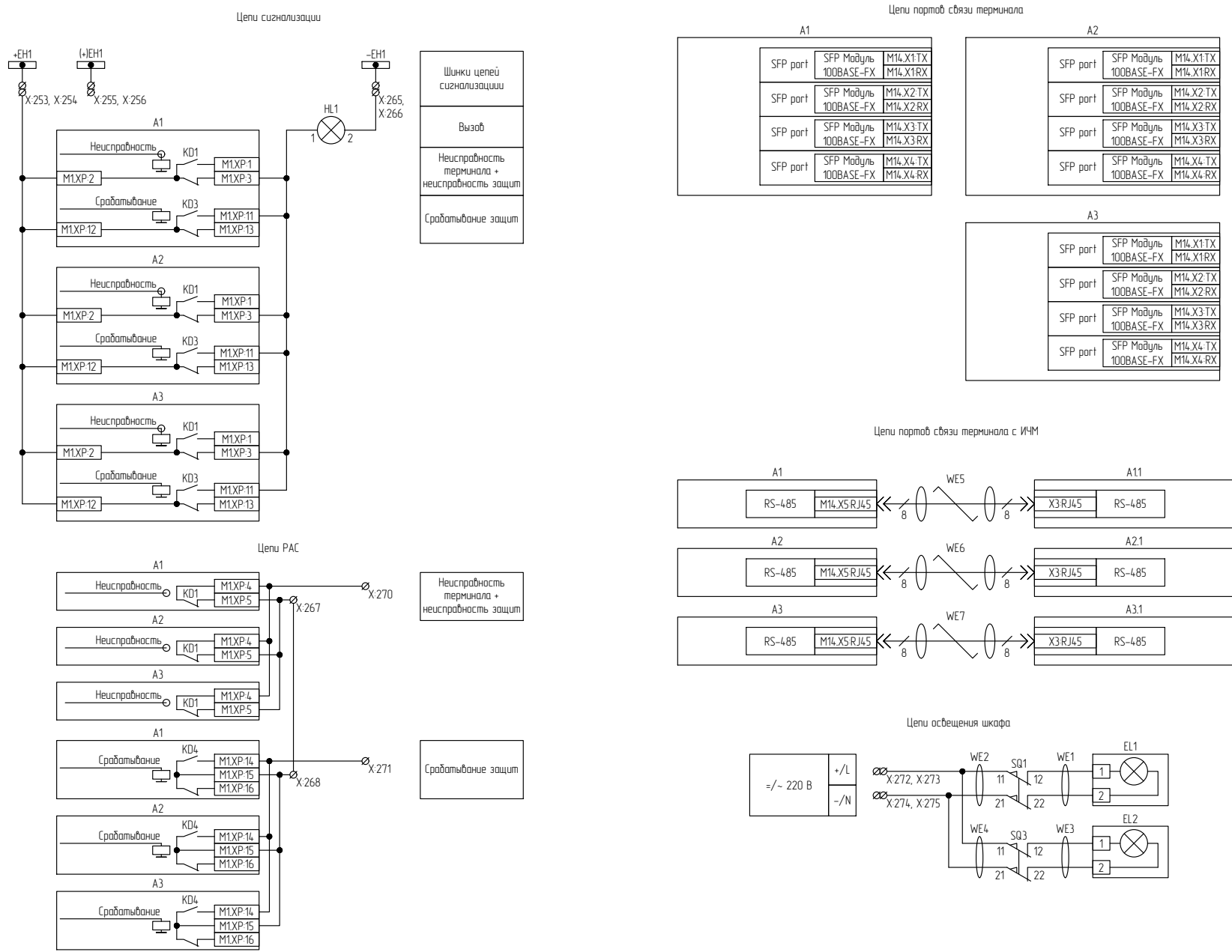
Рисунок В.8 – Схема электрическая принципиальная (часть 8)
