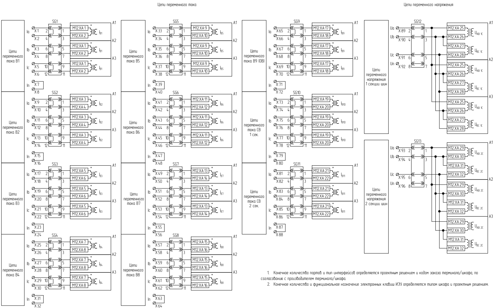
Рисунок В.1 – Схема электрическая принципиальная (часть 1)
