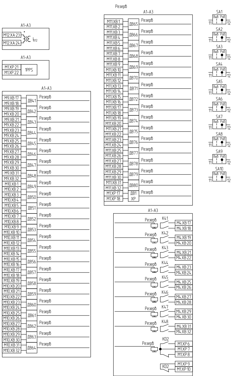
Рисунок В.9 – Схема электрическая принципиальная (часть 9)
